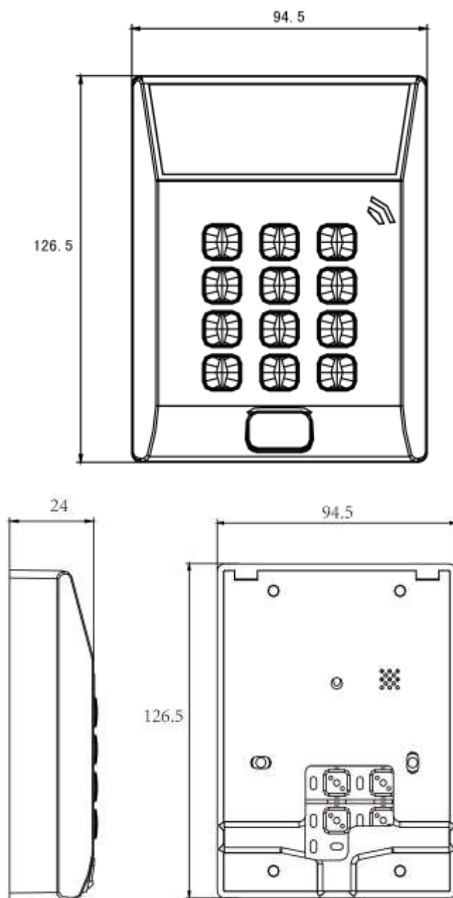
图2-1 DS-K1T802 外观尺寸
