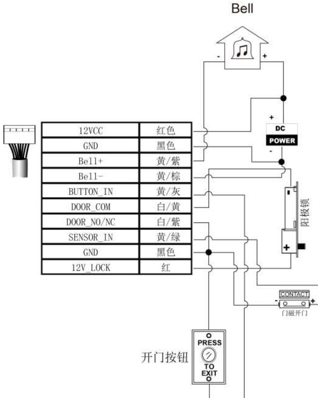
图3-1 一体机尾线示意图
