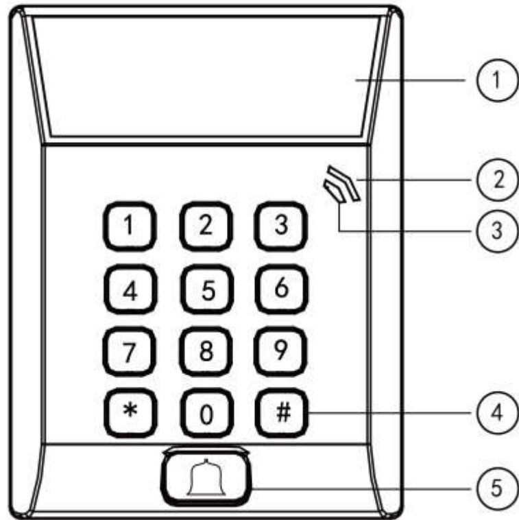
图2-2 DS-K1T802 外观说明
