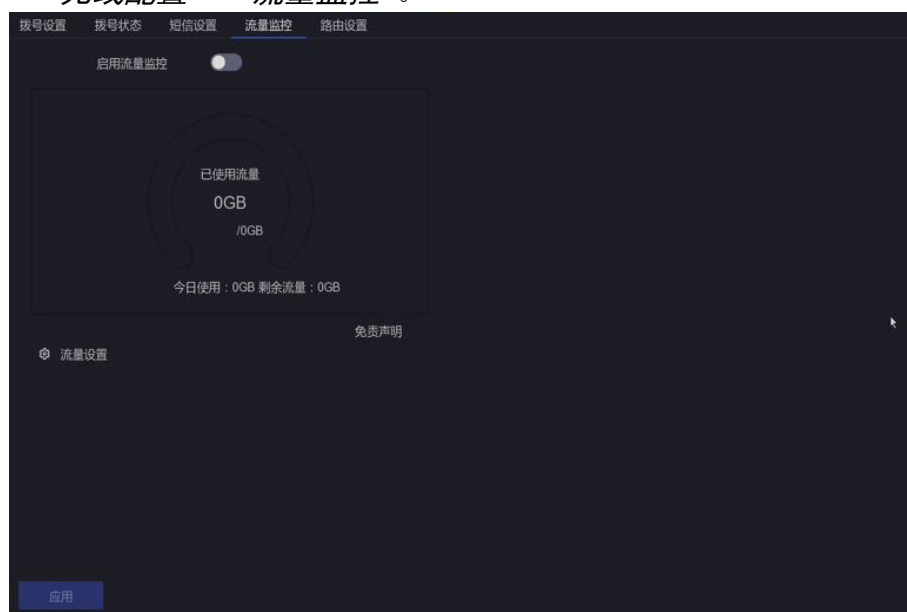
图 9-4 流量监控
