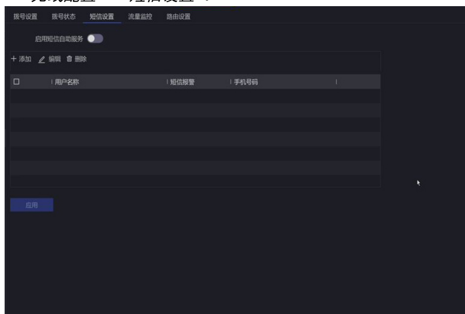
图 9-3 短信设置
