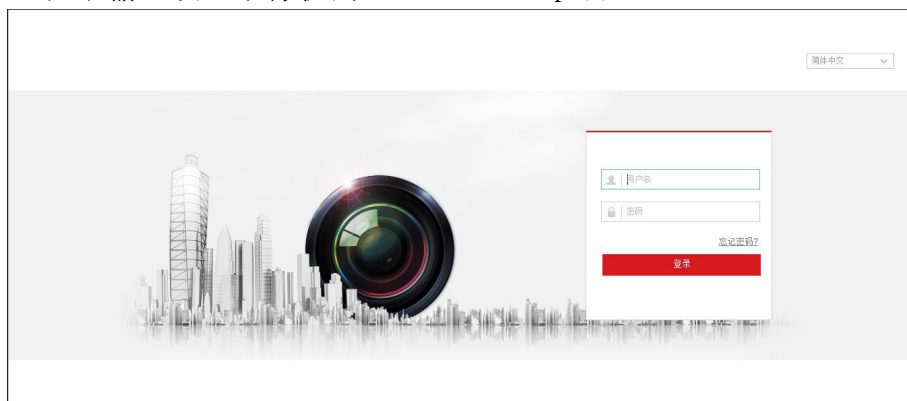
图 13-1 登录界面
