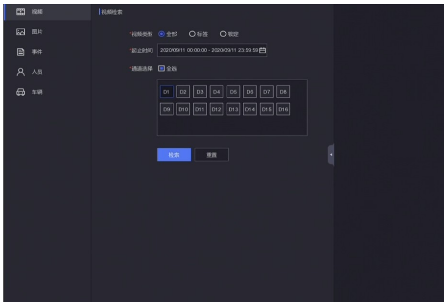
图 7-1 检索界面
