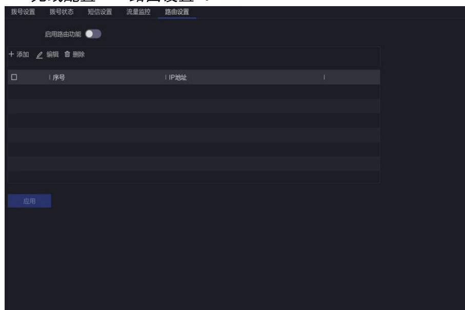
图 8-5 路由设置
