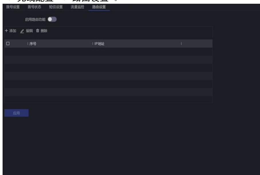
图 9-5 路由设置
