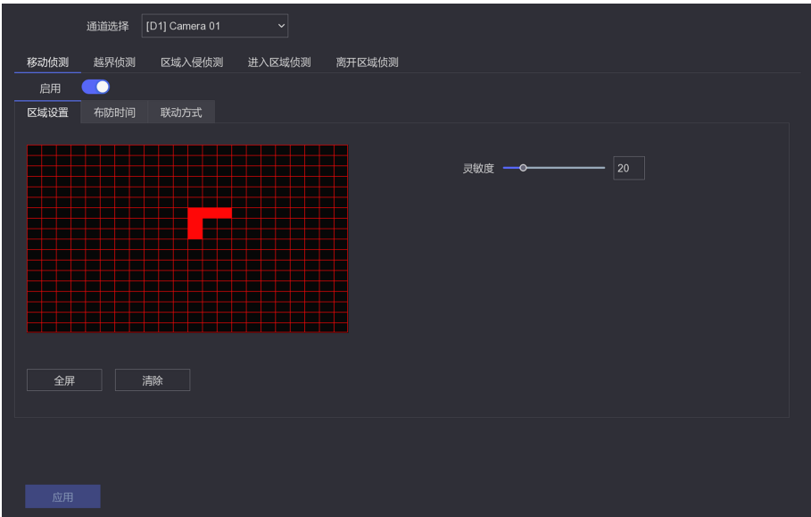
图 8-7 事件配置
