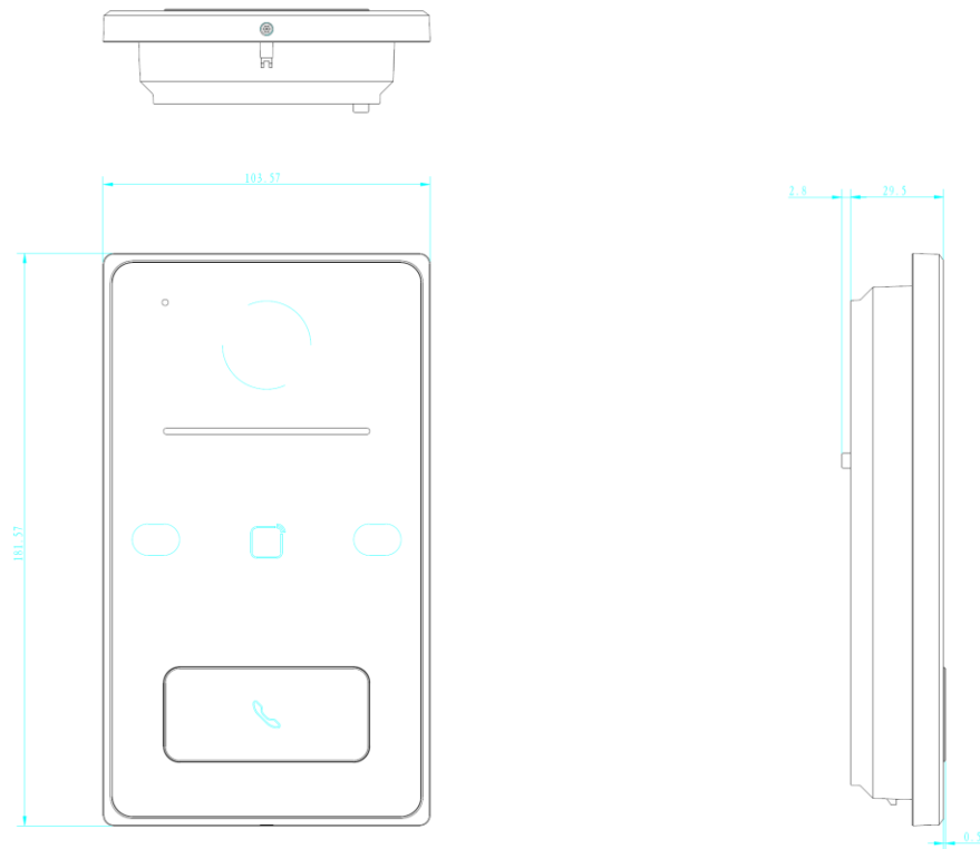
DS-KVJ133-M1 DS-KVJ133-MW1
